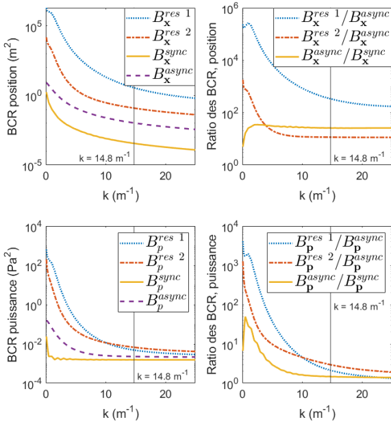
FIGURE 2 : Bornes de Cramér-Rao en position et en puissance dans le cas de réseaux parallèles avec 2 sources, pour les réseaux seuls, le cas synchrone et le cas asynchrone.
