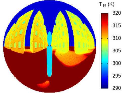
(d) Thermal environment without trees
