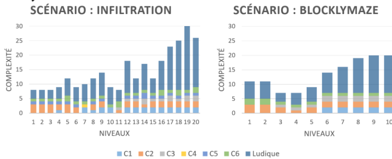
Fig. 2. Analyse des deux scénarios du jeu SPY
