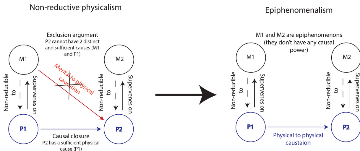
Fig. 3. The exclusion argument.
