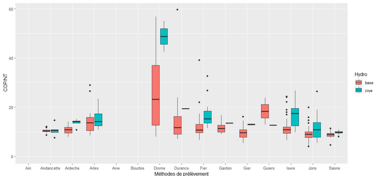
Figure 14. Boîtes à moustache des rapports C/N pour les différentes stations en fonction des conditions hydrologiques de base et de crue.
