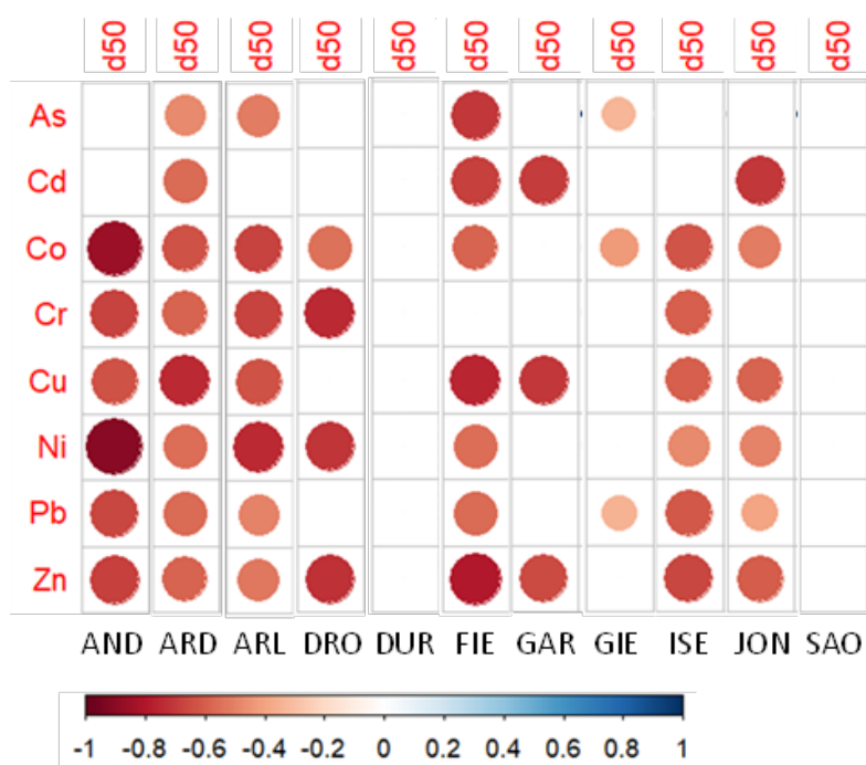
Figure 16. Corrélations (test de Pearson) obtenues entre la granulométrie (d50) et les concentrations en métaux (As, Cd, Co, Cr, Cu, Ni, Pb et Zn) pour les principaux affluents du Rhône (Ardèche, Drôme, Durance, Fier, Gardon, Gier, Isère et Saône). Les corrélations significatives ( p < 0.05 ) sont représentées par des ronds dont la couleur dépend du coefficient de corrélation (entre -1 pour la couleur rouge et +1 pour la couleur bleue).
