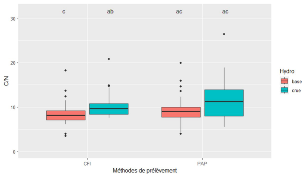
Figure 11. Boîtes à moustache des rapports en COP et NT (C/N) mesurés dans les MES prélevées à la station de Jons par centrifugation fixe (CFI) et par pièges à particules (PAP) lors de périodes hydrologiques de base (rose) ou crues (bleu).
