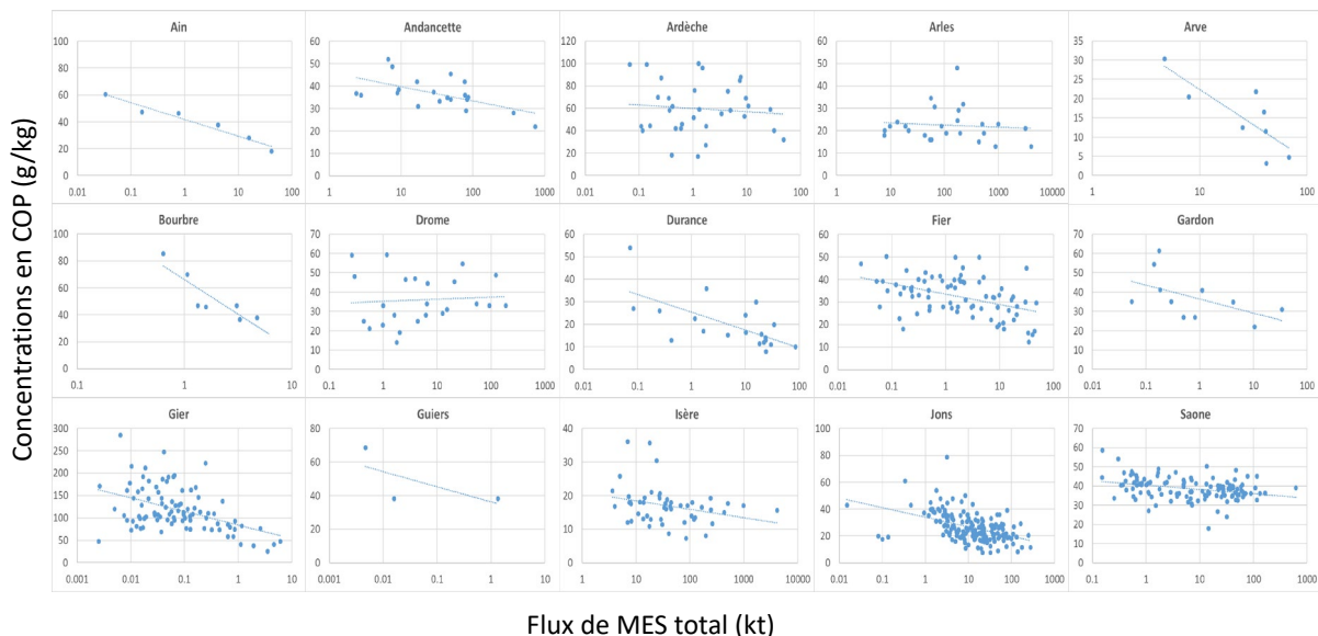
Figure 13. Variation des concentrations en COP en fonction des flux de MES pour les prélèvements par PAP au niveau des différentes stations. L'axe des flux est en logarithme base 10.
