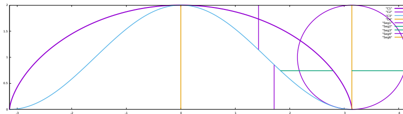
Figura 2: cicloide, compagna, ciclo generatore e indivisibili corrispondenti
