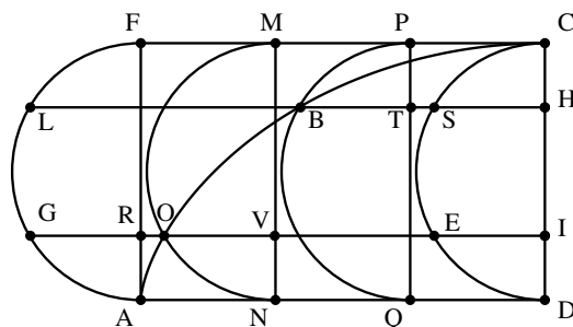
Figura 4: Torricelli: 'III dimostrazione', con metodo degli indivisibili
