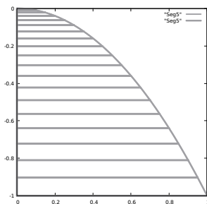
Figura 5: Roberval: parabola, metodo degli indivisibili
