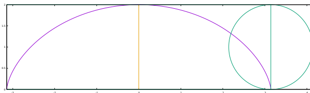
Figura 1: Cicloide, asse e cerchio generante (di raggio 1): il suo punto inizialmente in (\pi, 0) traccia, mentre il cerchio rotola senza strisciare, la curva cicloide. La semi-cicloide è la parte racchiusa nel rettangolo formato dalle due linee verticali, delle quali la prima è l'asse e l'altra segna il diametro del cerchio nella posizione iniziale.
