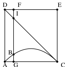
Figura 3: Torricelli: quadratura parabola, metodo degli indivisibili
