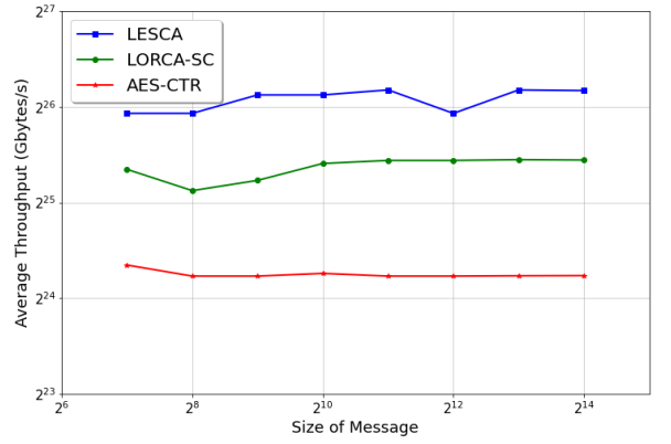
(d) Teensy 4
