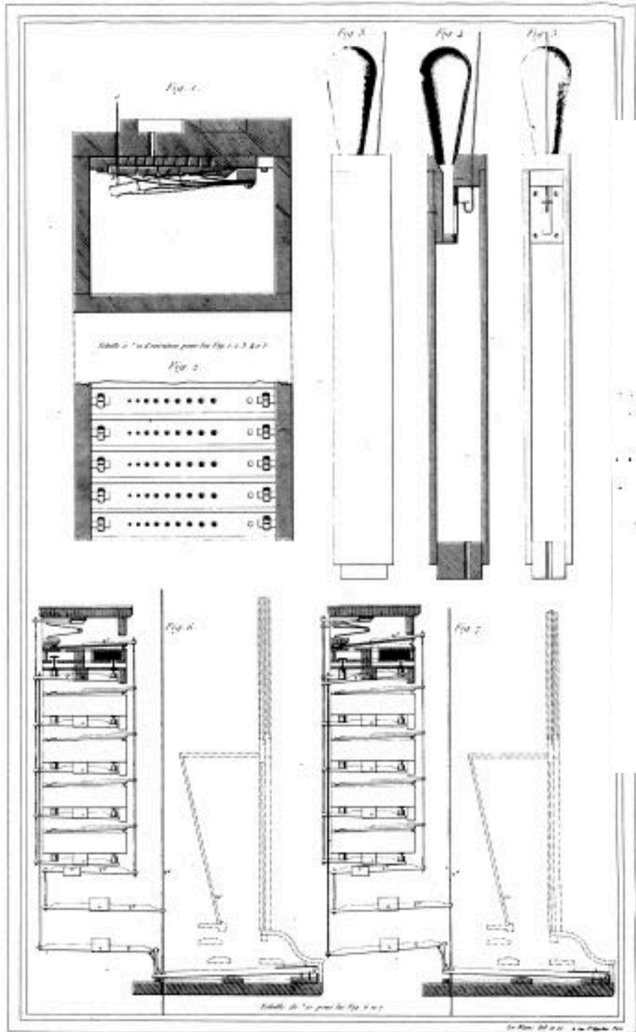
DÉTAILS ESSENTIELS ET CARACTÉRISTIQUES DE L'ORGUE DE LA CHAPELLE DES TUILERIES. DRESSÉ ET GRAVÉ PAR SÉBASTIEN ET PIERRE ÉRARD.
