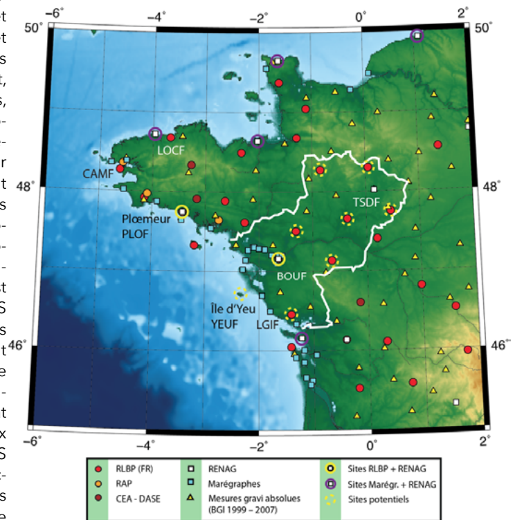
1. Carte des stations d'observation géophysique dans l'Ouest de la France métropolitaine. Sources : bgi.obs-mip.fr, refmar.shom.fr, renag.resif.fr, seismology.resif.fr, sonel.org
