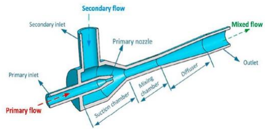
Fig. 2. Principe de la ligne d'hydrogène avec recirculation [15] et de l'éjecteur [16].
