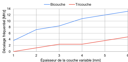
Figure 8. Décalage fréquentiel simulé en fonction de l'épaisseur de la couche externe (graisse pour la bicouche et muscle pour la tricouche)
