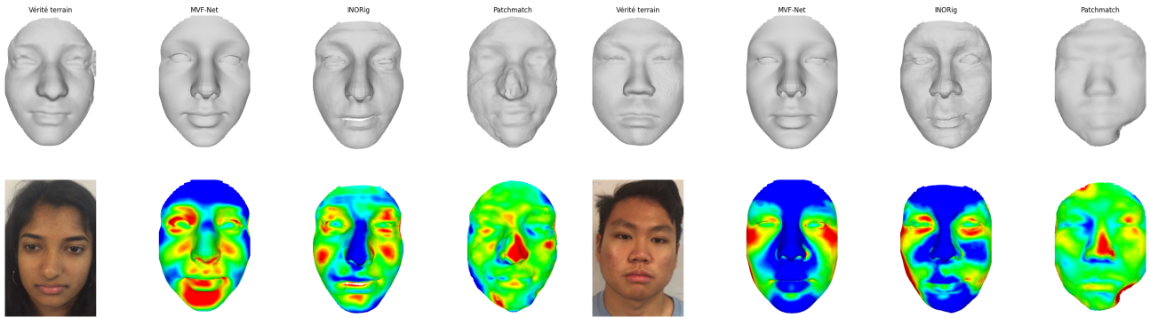
FIGURE 3 – Résultats sur deux exemples de 3DFAW-vidéo, l’erreur est signée, l’échelle va de -3\text{mm} (rouge) à 3\text{mm} (bleu)
