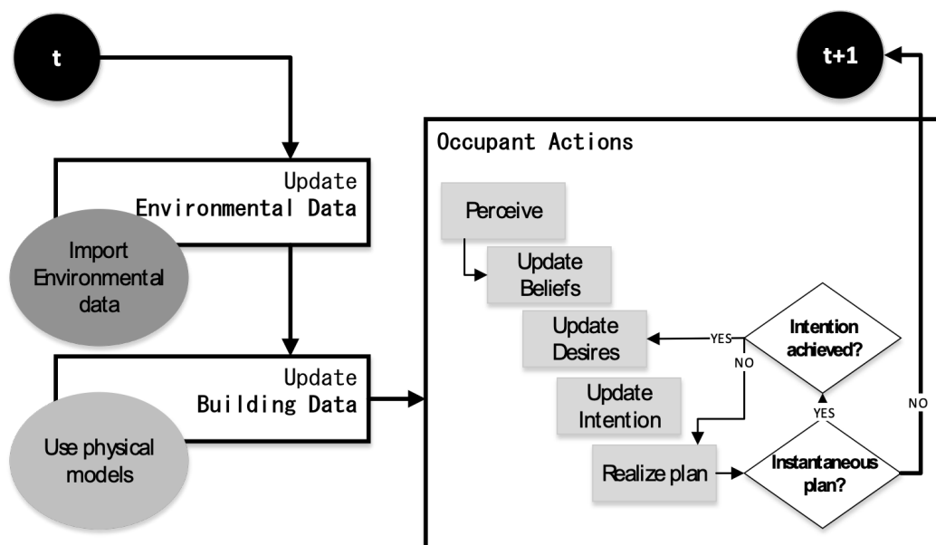
FIGURE 4. Dynamique de Li-BIM (Micolier et al., 2019)
