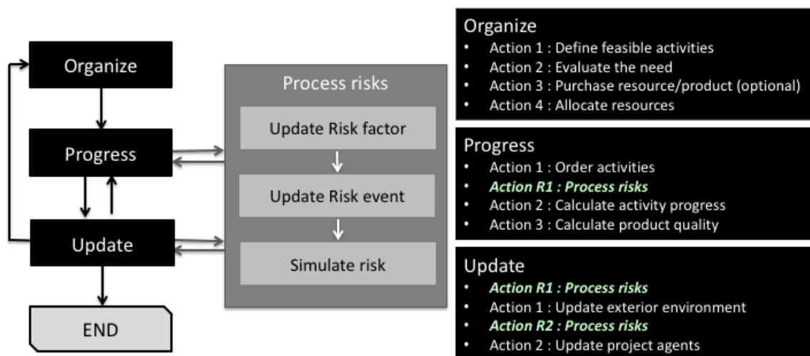
FIGURE 3. Dynamiques dans SMACC2 (Taillandier et al., 2016)
