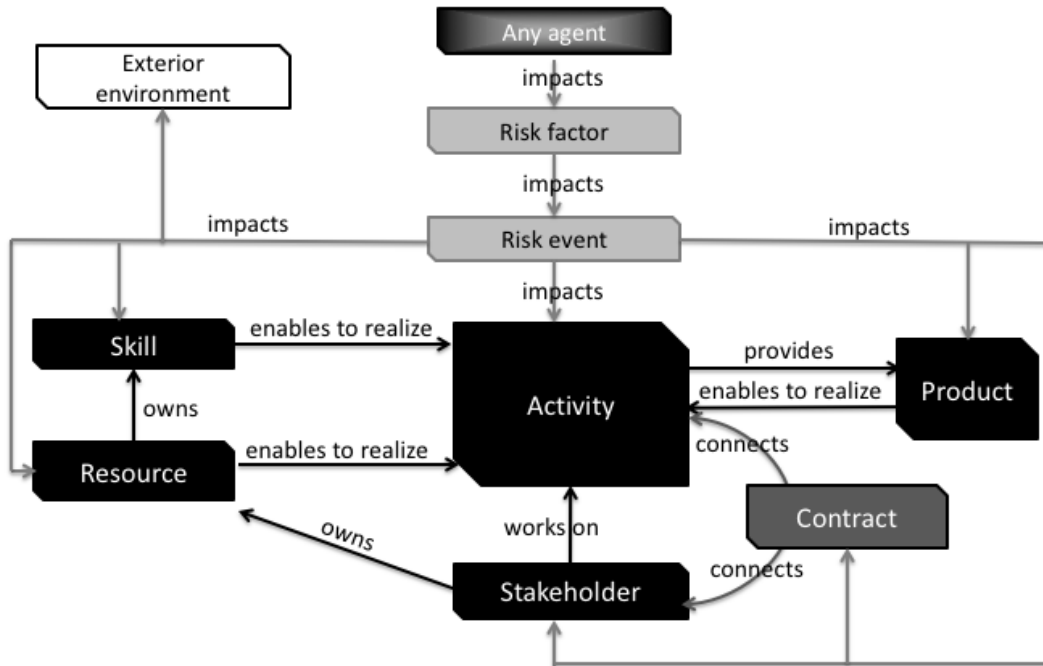
FIGURE 2. Agents dans SMACC2 (Taillandier et al., 2016)
