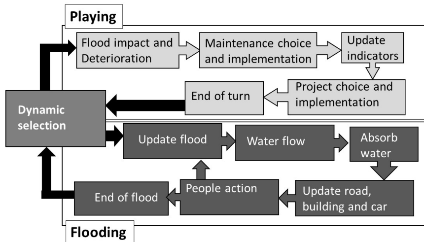
FIGURE 7. Dynamiques de MANA-Flo (Taillandier et al., 2022)
