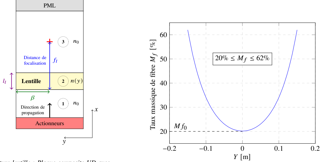
(a) Structure lentille : Plaque composite UD avec une lentille à gradient d'indice de réfraction ; avec \vec{x} la direction des fibres ; zone ② : M_f = M_f(y) ; zones ① et ③ : M_f = M_{f_0}
