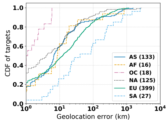
Figure 4: Error per continent
