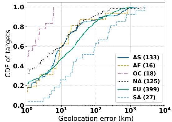
Figure 4: Error per continent
