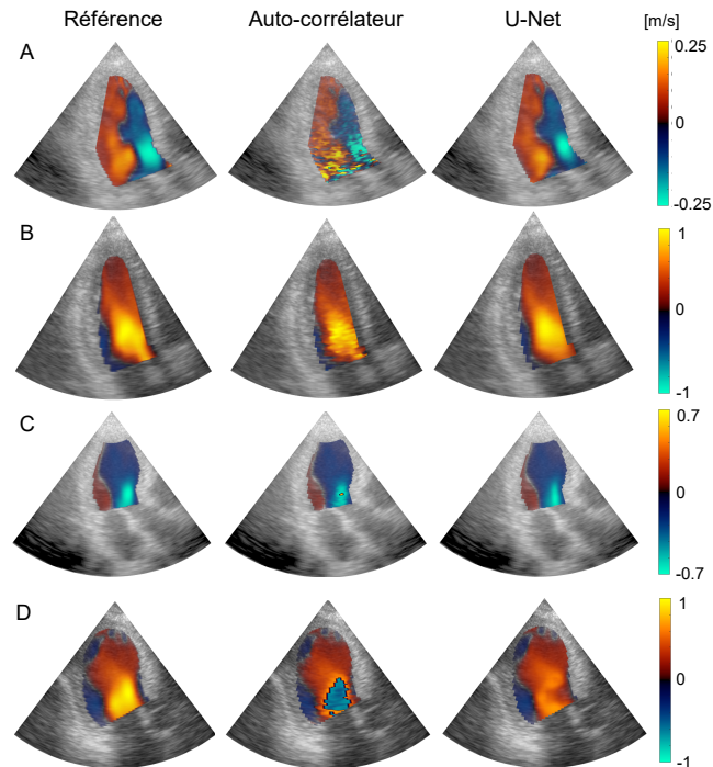
FIGURE 1 : Exemples de références de vitesses Doppler et des vitesses estimées par l’autocorrélateur et le U-Net pour des packet size de n = 2 . Les champs de vitesses sont superposés sur les images B-mode simulées correspondantes. (A) Exemple de cas avec un bruit gaussien de 25 dB. (B) Exemple de cas de surlissage du U-Net. (C) Exemple de cas avec une petite région avec du repliement. (D) Exemple de cas avec une grande région avec du repliement.
