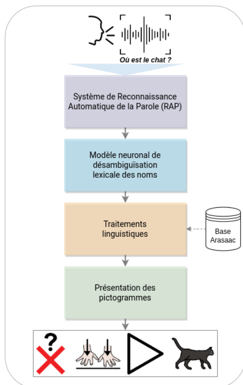
FIGURE 1 – Schéma de Voice2Picto.
