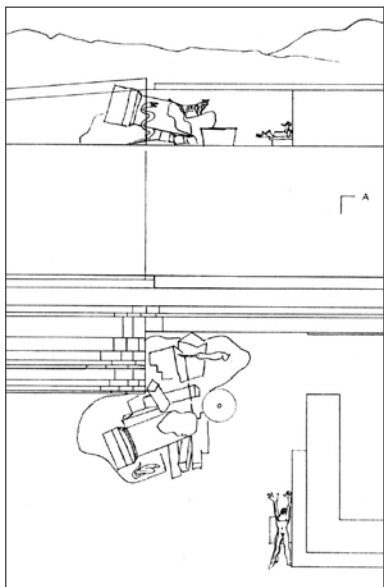
Figure 15. Vue en plan et élévation du « tumulus » et du gisant (détail) (JEANNERET, C. E. – LE CORBUSIER, dans Boesiger, 1965).
