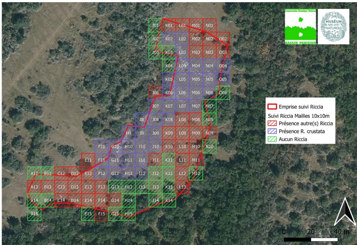
Figure 27 : Résultat du suivi des Riccia en 2021. Les mailles à Riccia crustata sont en violet.
