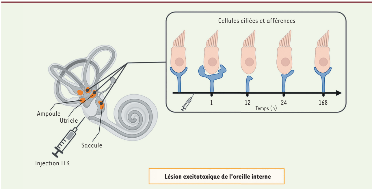
Figure 3. Injection de TTK et lésion excitotoxique de l'oreille interne. L'injection d'acide kainique (TTK) entraîne une souffrance des afférences primaires au contact des cellules ciliées vestibulaires situées dans les organes otolithiques (sacculle, utricule) et les ampoules selon une temporalité précise. Les terminaisons nerveuses afférentes gonflent (1 heure après injection), entraînant leur résorption (7-12 heures après injection) suivie d'une réparation (à compter d'une semaine après la lésion). L'altération de la zone de contact entre cellules ciliées vestibulaires de l'oreille interne et afférences (bleu) formant le nerf vestibulaire engendre un syndrome vestibulaire transitoire (figure créée avec Biorender.com).
