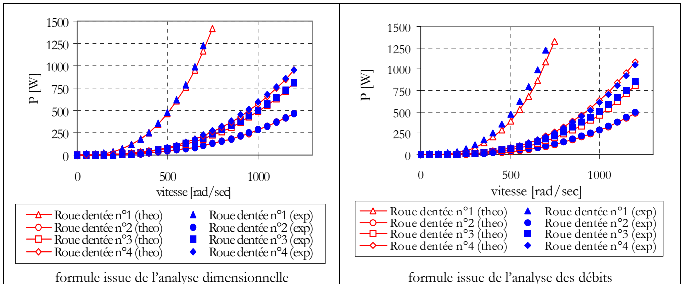
FIG. 3 – Comparaisons entre les résultats expérimentaux et les différents modèles.
