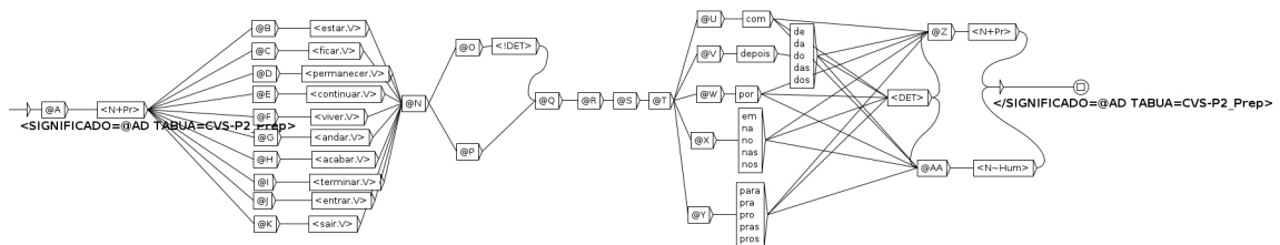
Figura 3. Grafo parametrizado para CVS-P2_Prep
