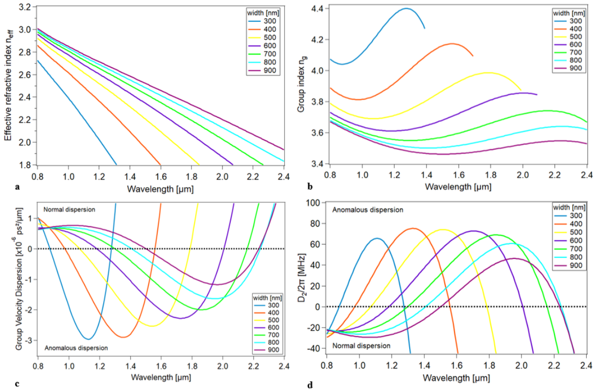
Figure 2: Simulation par éléments finis pour un microrésonateur en anneau de 300 nm de GaP sur \text{SiO}_2 avec différentes largeurs de guide w pour le mode TE_{00} . (a) Indice de réfraction effectif n_{eff} en fonction de \lambda . (b) Indice de groupe n_g en fonction de \lambda . (c) GVD en fonction de \lambda . (d) Paramètre de dispersion en fonction de \lambda .
