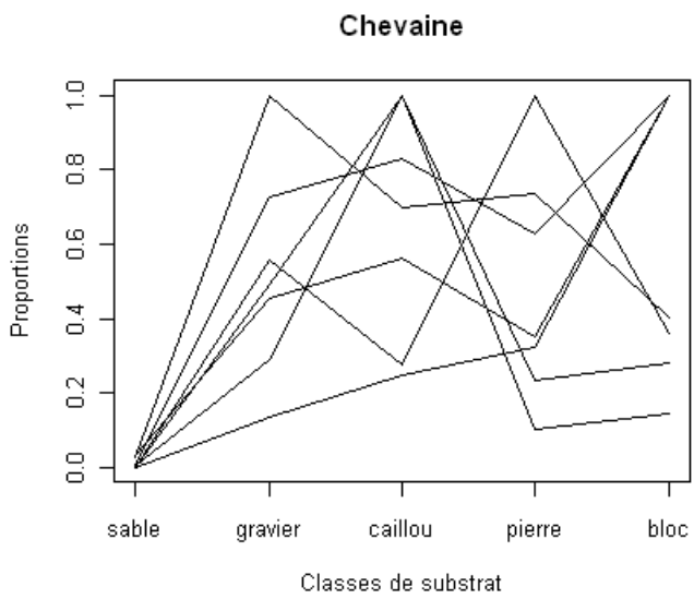
Figure 38 : courbes de préférences des 7 chevaines les mieux suivis pour chacune des 4 variables physiques retenues (profondeur, vitesse du courant, substrat et température de l'eau).
