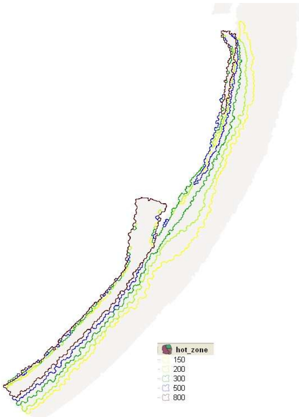
Figure 24 : contour du panache d'eau chaude simulé pour 150, 200, 300, 500 et 800 \text{m}^3.\text{s}^{-1} . Physiquement il n'existe pas de limite stricte, mais un gradient de température (diffusion) au contact entre les veines d'eau chaudes et froides. Nous avons choisi comme limite, les nœuds du maillage pour lesquels la température simulée était de 2°C plus élevées que la température à l'amont du site. Ce sont les contours des aires d'influence de ces nœuds ayant une température plus chaude de 2°C, qui forment les contours présentés sur cette figure.
