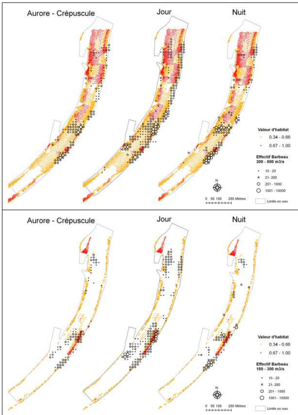
Figure 43 : Cartographie des VH aux nœuds du maillage du modèle hydrodynamique calculées avec les courbes de préférence du barbeau adulte de Lamouroux et al. (1999) en haut (à débit moyen) et avec les hydrosignatures de préférence (profondeur * vitesse) de notre étude de 2009 en bas (à débit faible). Les localisations des barbeaux suivis en 2009 sont superposées en fonction des phases nyctémérales et représentées en 4 classes de nombre de localisation par carreau de la grille à 20 m. (les simulations ont été réalisées pour les trois classes de débit, mais seuls deux exemples sont montrés ici).
