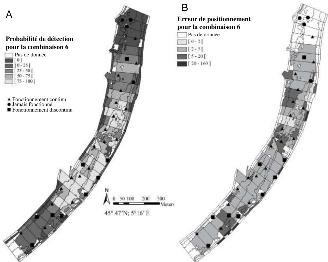
Figure 31 : Cartes de probabilité de détection et carte d'erreur de positionnement générées pour la combinaison de variables qui permet d'obtenir la meilleure précision. (d'après Bergé et al. , 2012).
