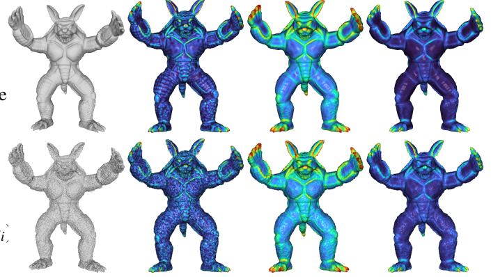
FIGURE 2 – Robustesse au bruit. Maillage original (haut) et bruité (bas) avec leurs rugosité, saillances géométrique et spectrale (de gauche à droite) sur des 3-ring avec des descripteurs 2-hop en spirale.
