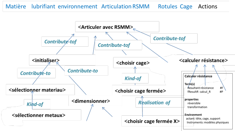
FIG. 3 – Une sous-ensemble de l'ontologie des actions
