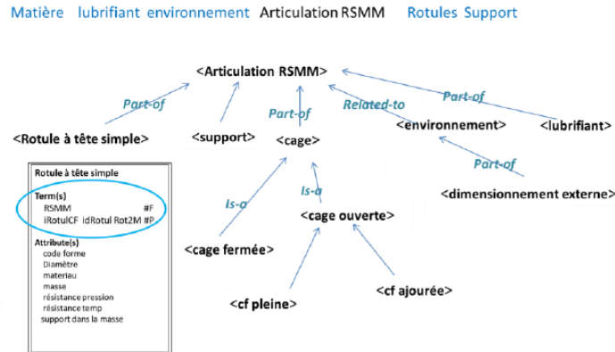
FIG. 2 – Extrait de l'ontoterminologie métier et correspondance avec le code
