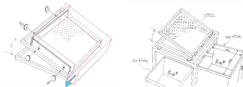
Figure 2 : Schémas du nouveau bâti d'essai de perméabilité
