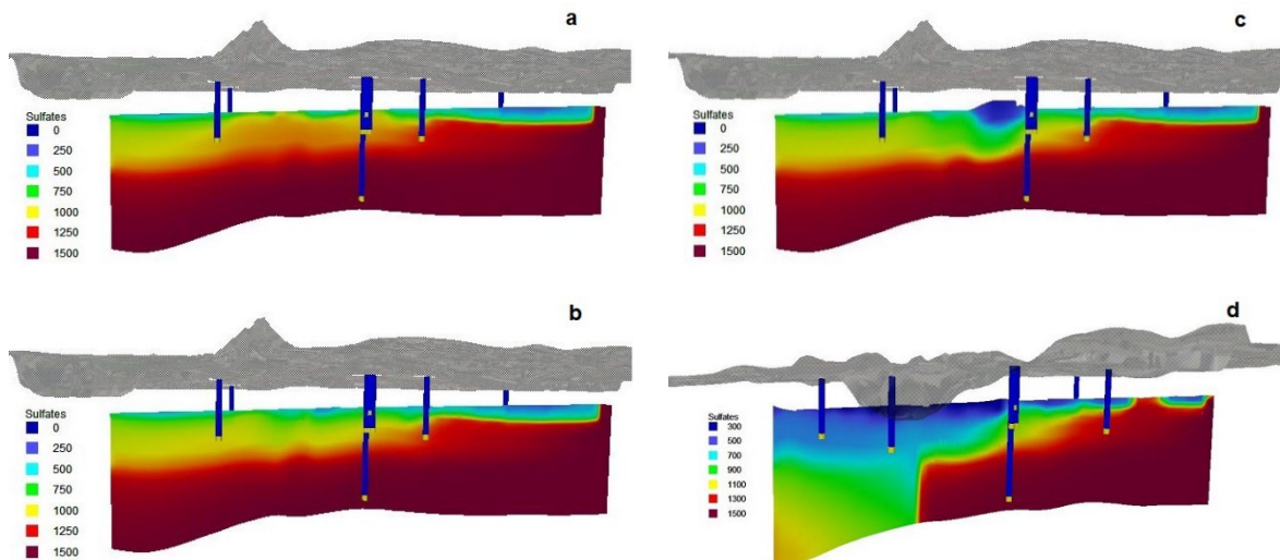
Figure 2 : Profil des concentrations (mg/L) simulées pour l'état actuel (a), le scénario de gestion diffuse (b), le scénario de gestion centralisée (c) et le scénario de gestion centralisée avec la présence d'une discontinuité (d)
