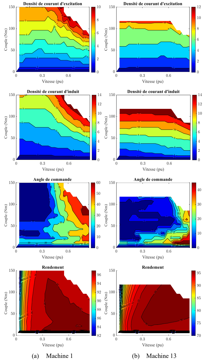
Fig.9. Cartographies de deux machines issues de l'optimisation sur cycle.
