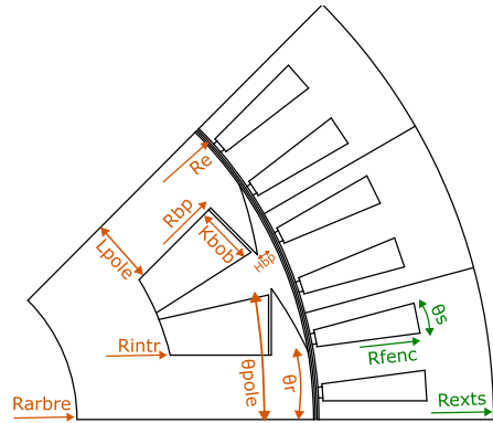
Fig. 6. Modèle paramétrique de la MSRB.
