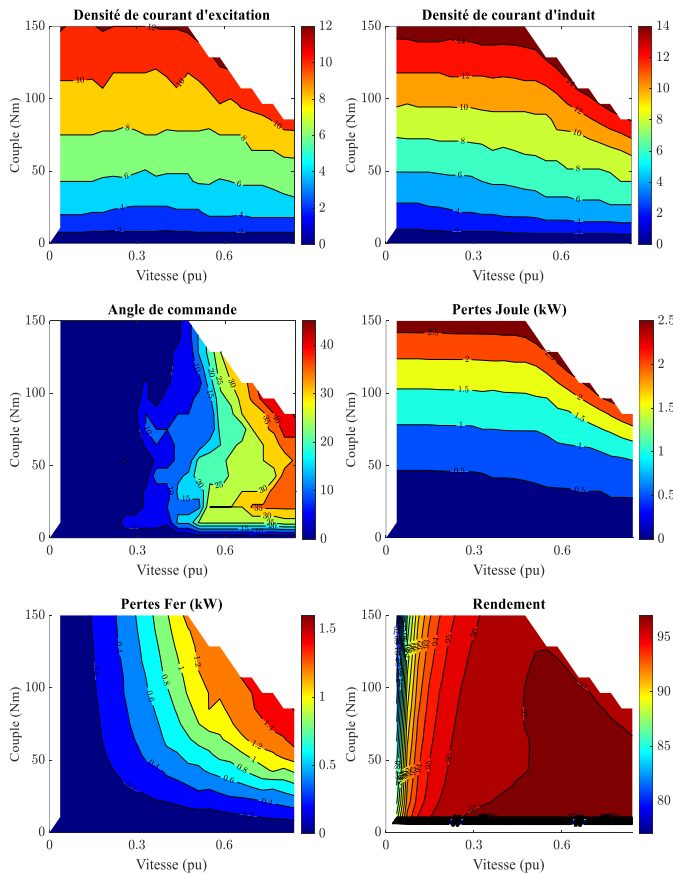
Fig. 5. Cartographies obtenues à l'issue des calculs sur cycle.
