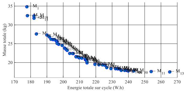
Fig. 7. Front de Pareto des résultats d'optimisation.
