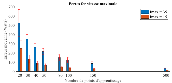
Fig. 2. Évolution de l'erreur en fonction du nombre de points d'apprentissage.
