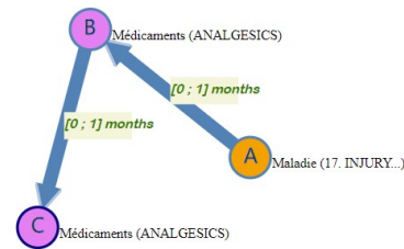
FIG. 5 – Chronique avec des évènements multiples et des délais.
