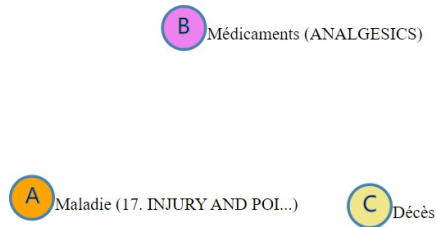
FIG. 4 – Chronique avec des évènements multiples.
