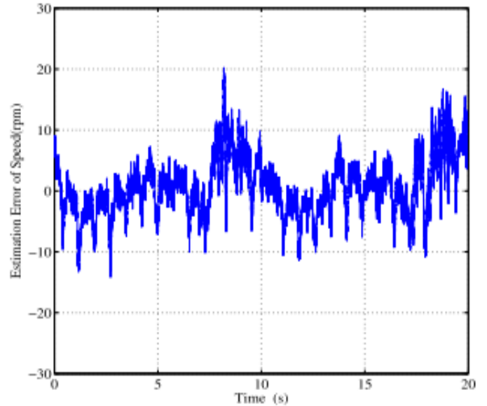
Fig.6. Variation de l'erreur d'estimation de la vitesse
