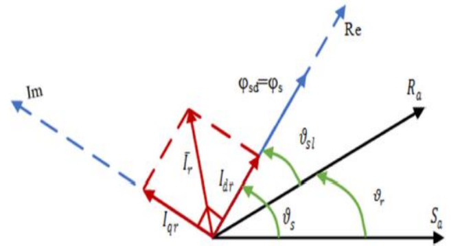
Fig.1. Orientation du Flux Statorique.
