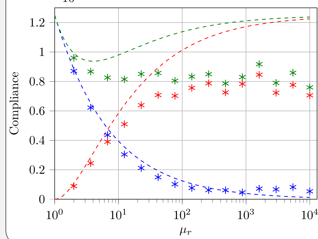
Fig. 6 : Compliances en fonction de \mu_r (linéaire)
