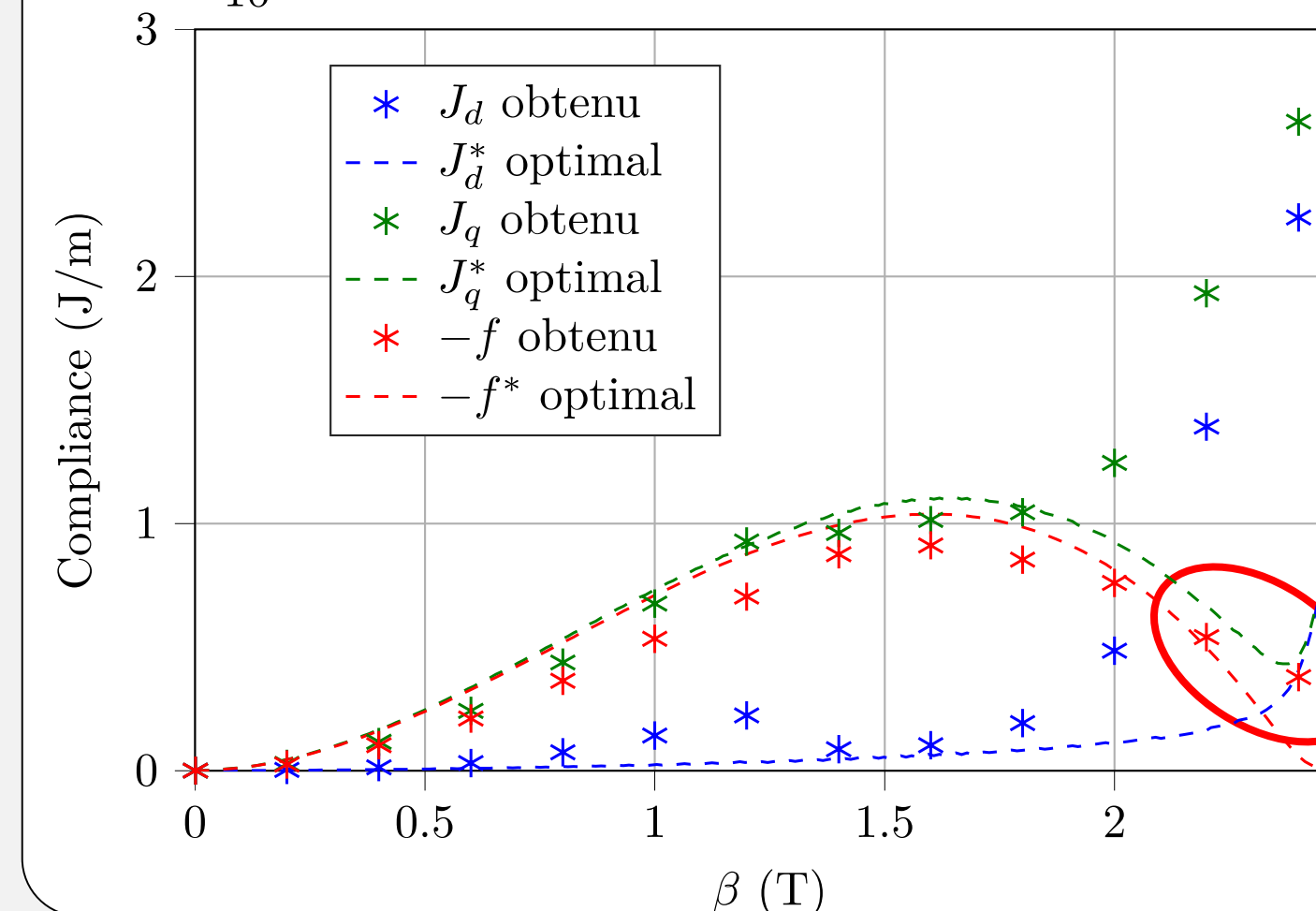
Fig. 11 : Compliances en fonction de \beta (non-linéaire)
