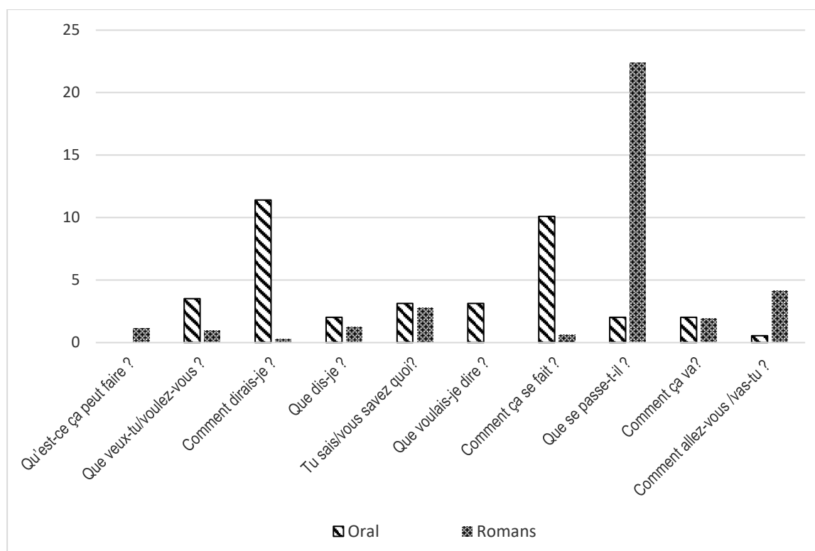
Figure 3 : Distribution des PIPP (toutes variantes syntaxiques) selon les 2 corpus (en fréquence relative, pour 1 million de tokens)
