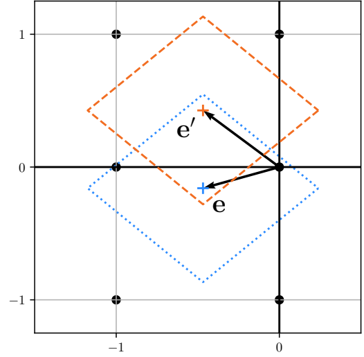
FIGURE 2 : Exemple jouet avec des blocs de taille (1, 2) . Le vecteur \mathbf{e} est l'erreur d'arrondi spatial d'un bloc cover et \mathbf{e}' est l'erreur d'arrondi spatial du même bloc après avoir inséré un message stego dedans. Le carré en pointillés bleus et le carré en tirets oranges représentent les contraintes de l'ensemble des erreurs de compression possible \mathcal{S} dans chacun des cas. Notez qu'il n'y a aucun point de coordonnées entières dans le carré en tirets oranges prouvant que ce bloc est incompatible.
