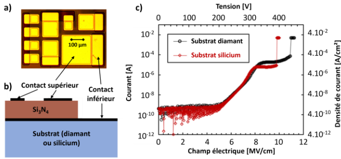
Figure 10 : Premiers essais de dépôts \text{Si}_3\text{N}_4 . a) Image en microscopie optique des capacités MIM sur substrat diamant. b) vue en coupe de la structure des capacités MIM. c) Mesure expérimentale du claquage.
