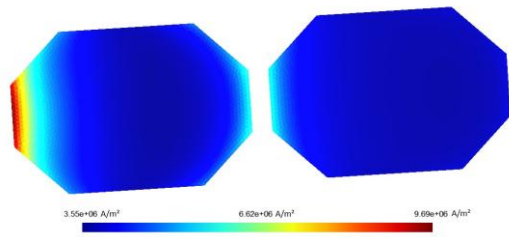
Fig. 7. Densité de courant dans une encoche (25 Nm, 5500 tr/min)
