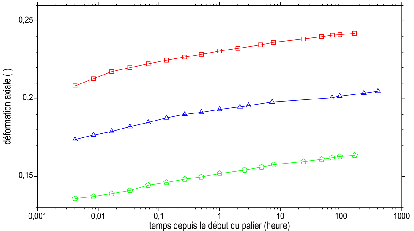
Courbes contraintes déformations et déformation temps.
