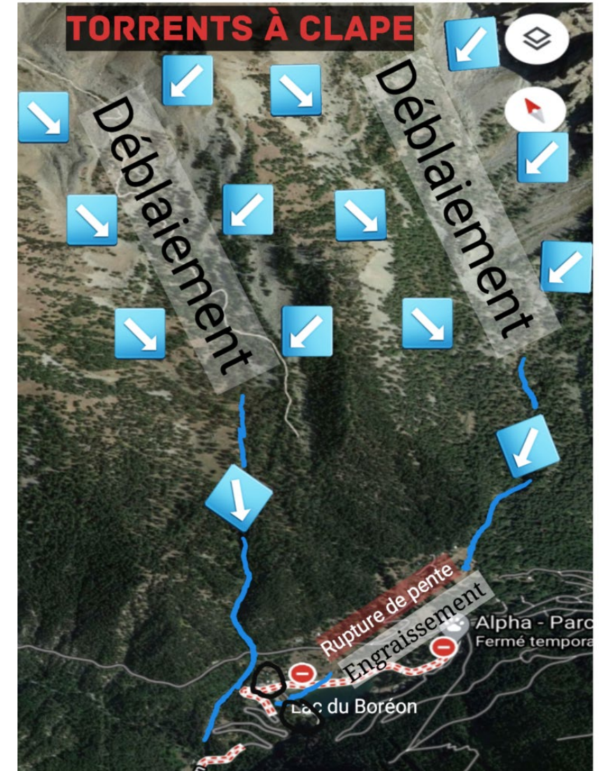
L'apport des des torrents à clape et torrents de laves en amont du lac du Boréon sur la commune de St Martin Vésubie (Source : BERTHET, 2020)
