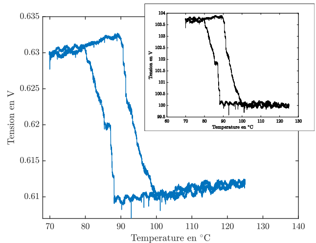
FIG. 5. Hystérésis thermique obtenue par mesure de réflectivité optique. Signal décimé de 100, après filtrage avec Butterworth d'ordre 4 et de fréquence de coupure 100 Hz. La courbe encadrée représente la même expérience avec des valeurs normalisée par rapport à la tension de la phase ferromagnétique (et multipliée par 100) afin de montrer la différence de réflectivité entre les deux phases. On remarque bien que la différence de réflectivité est de 3 à 4 % entre les deux phases
