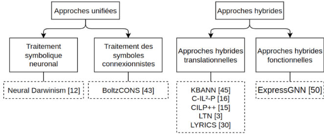
Figure 2. Illustration de la classification d'Hilario, adaptée de [20]. La seconde classification présentée ici est celle proposée en 2020 par Calegari et al. [4]. Les différents modèles sont triés selon leur type d'interprétabilité. Cette classification est illustrée par la figure 3.
