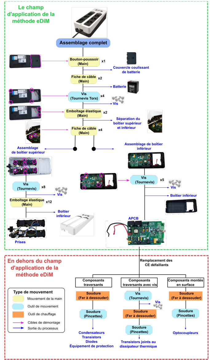
Fig.2. Séquence de démontage de l'onduleur.
