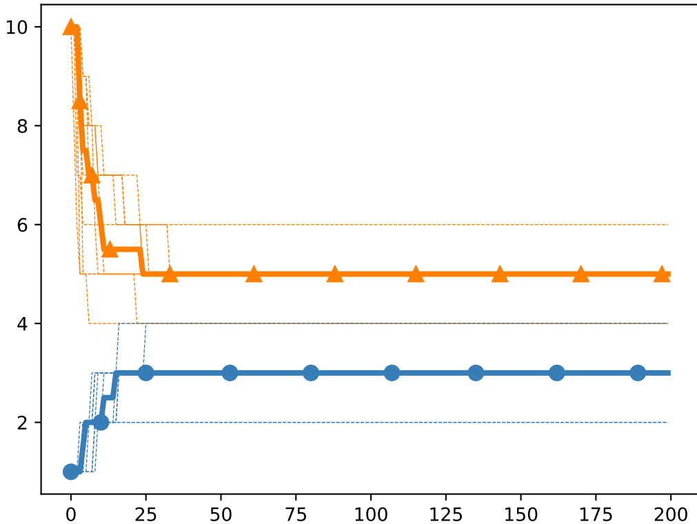
Chi Square mu:4.00, c:0.1, delta:0.05
