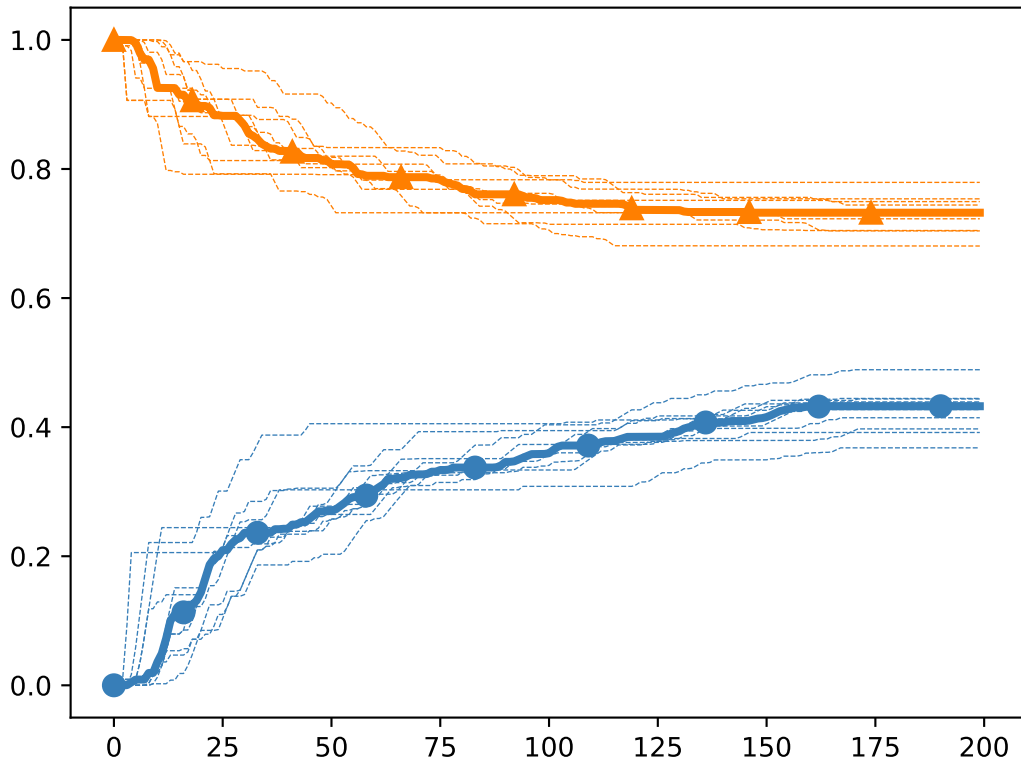
Bernoulli mu:0.57, c:0.1, delta:0.01
