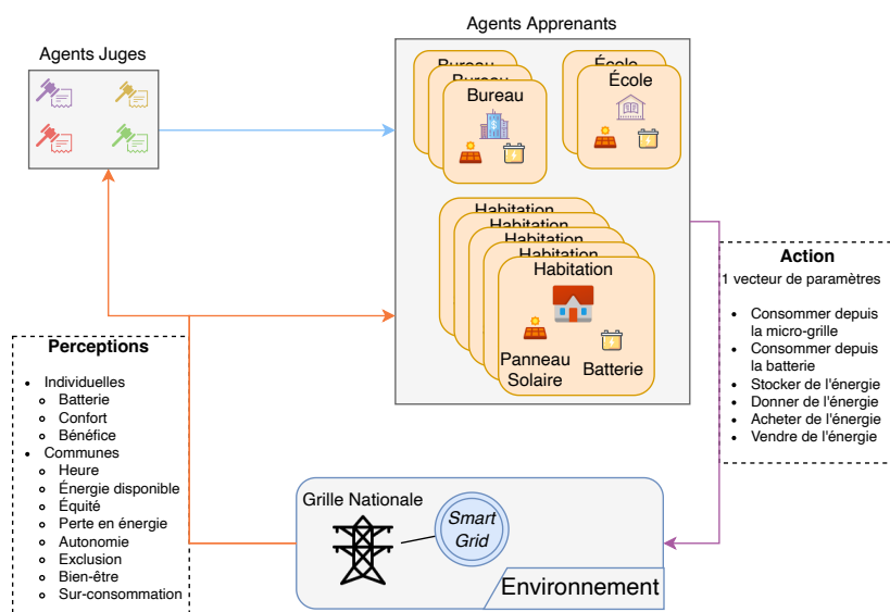
FIGURE 4.1. Schéma du simulateur de Smart Grid . Une micro-grille, liée à la grille nationale, contient plusieurs agents représentant des bâtiments.
