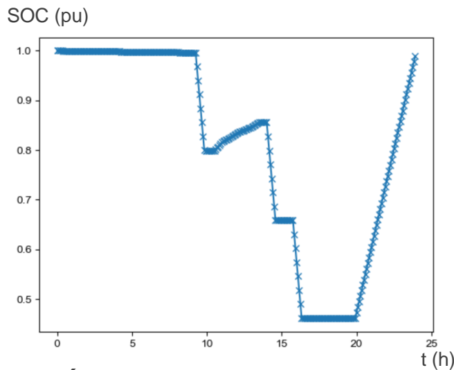
État de charge batterie sur une journée
