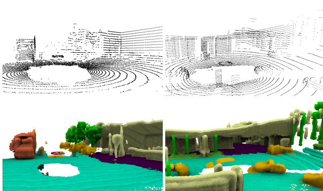
(b) nuScenes
