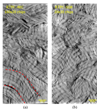
FIG. 3. – Comparaison des microstructures des matériaux recyclés à partir de différentes longueurs de fragments ((a) 160x20 mm et (b) 20x20mm) ; la structure initiale des fragments a été mieux conservée pour l'échantillon RTPC-SQR (b), tandis que plusieurs fragments semblent être déformés pour l'échantillon RTPC-REC (a).
