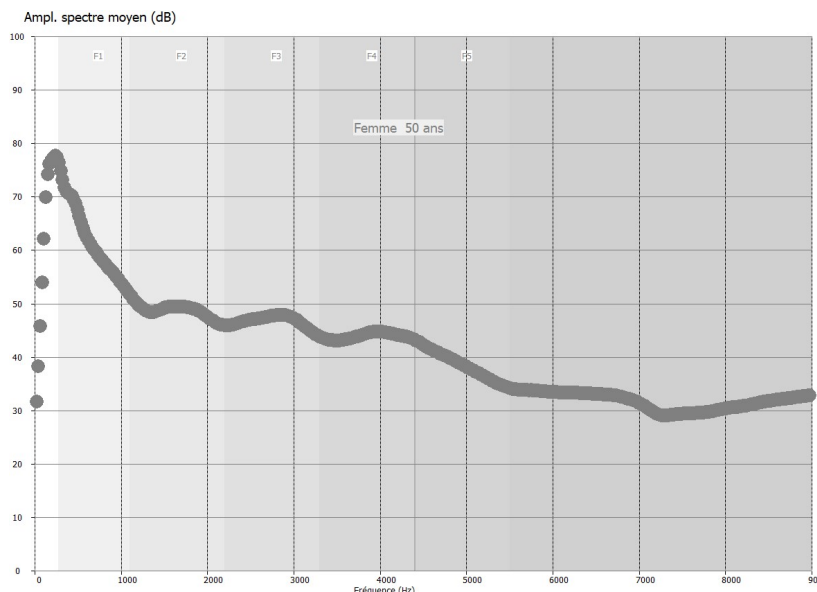
Figure 9 : Spectre moyen de la parole cumulé de 60 femmes
